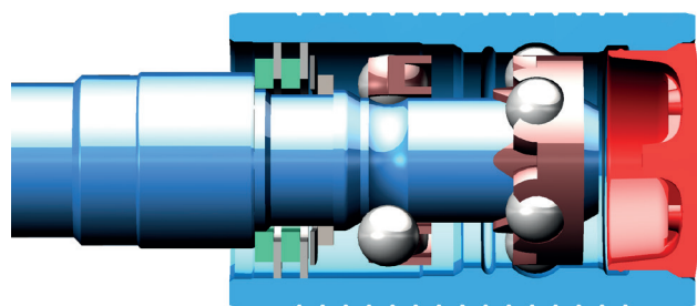
微密封系统的剖视图
